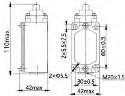
YBLX-K3 Dimensions
